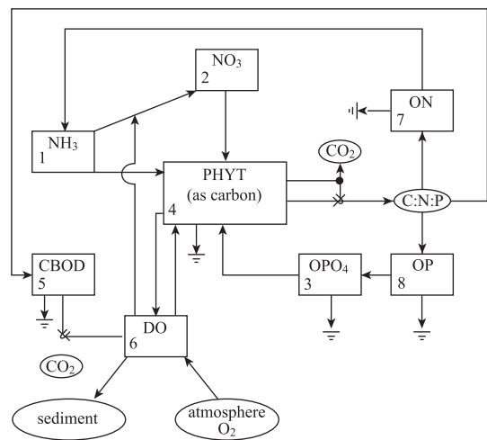
圖 2 水質模式 WASP 模擬水質項關係圖
