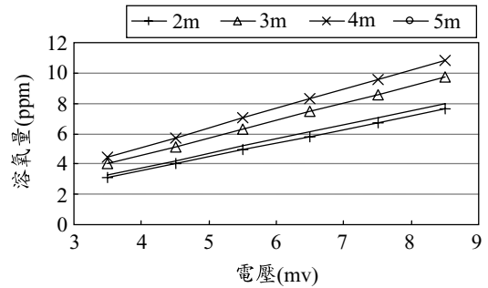
圖 3 不同導線長度之感應電壓強度與溶氧量關係圖
