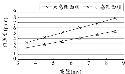
圖 6 不同感測面積之感應電壓強度與溶氧量關係圖
