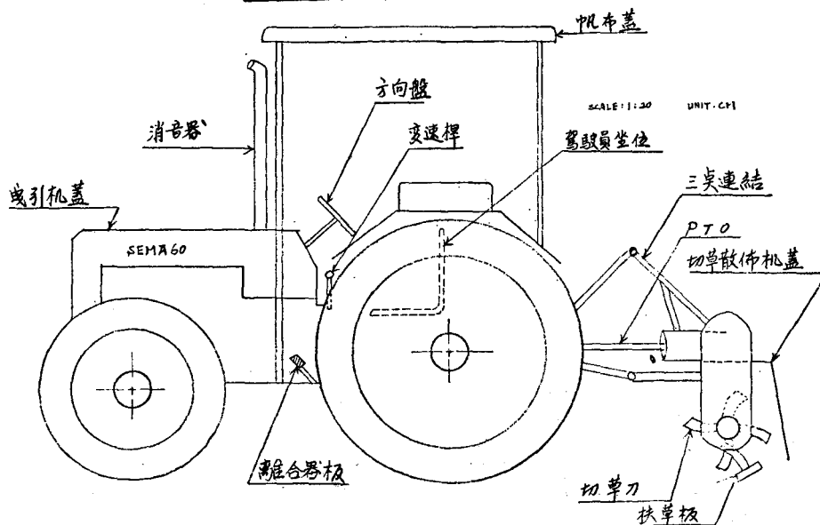
圖一 曳引機附裝切草散佈機側面圖
