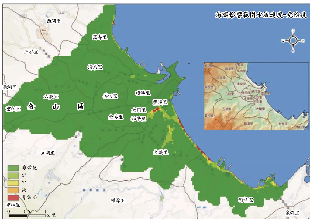
圖 12 新北市金山與萬里區海嘯影響範圍水流速度-危險度空間分布圖
