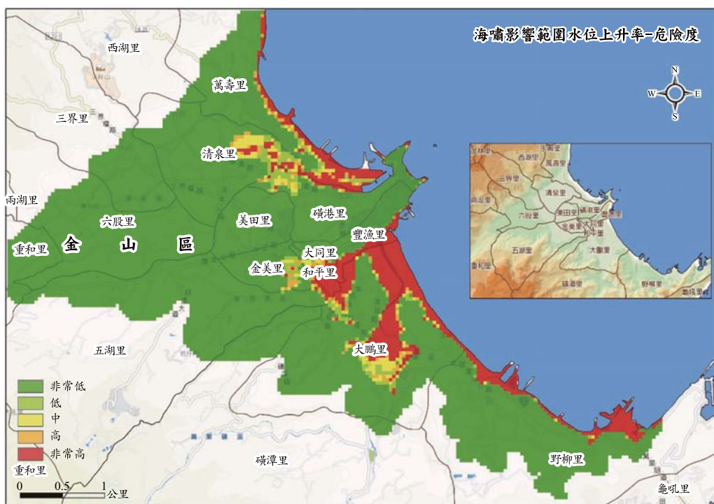
圖 13 新北市金山與萬里區海嘯影響範圍水位上升率-危險度空間分布圖
