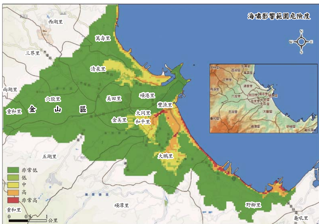
圖 14 新北市金山與萬里區海嘯影響範圍危險度空間分布圖(權重 \alpha_1 、 \beta_1 、 \gamma_1 各為 1/3)
